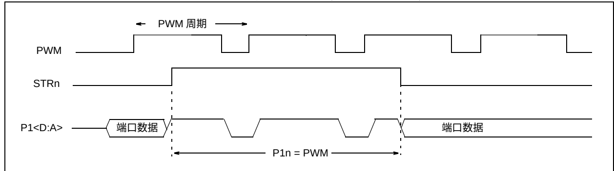
图 11-19： 指令结束时发生的转向事件的示例 (STRSYNC = 0)
