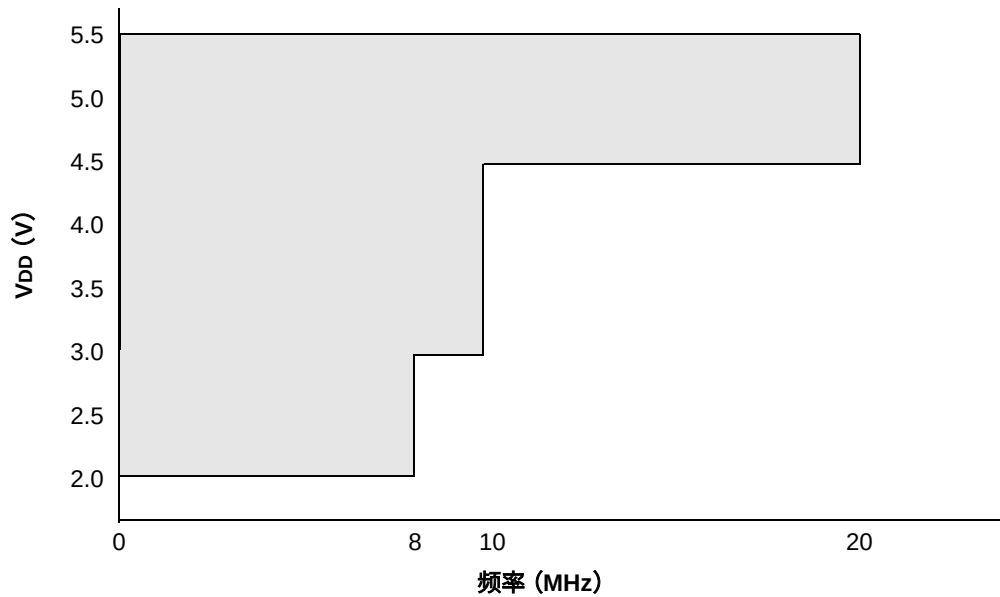
图 17-1： PIC16F631/677/685/687/689/690 电压—频率关系图， -40^{\circ}\text{C} \leq T_A \leq +125^{\circ}\text{C}
