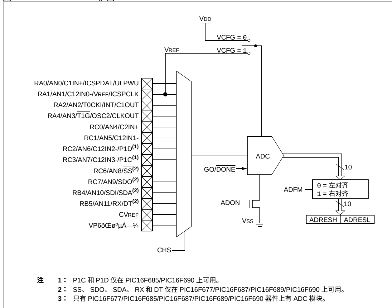
图 9-1： ADC 框图
