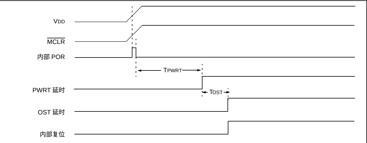
图 14-6：上电时的延时时序（带有 VDD 的 MCLR）
