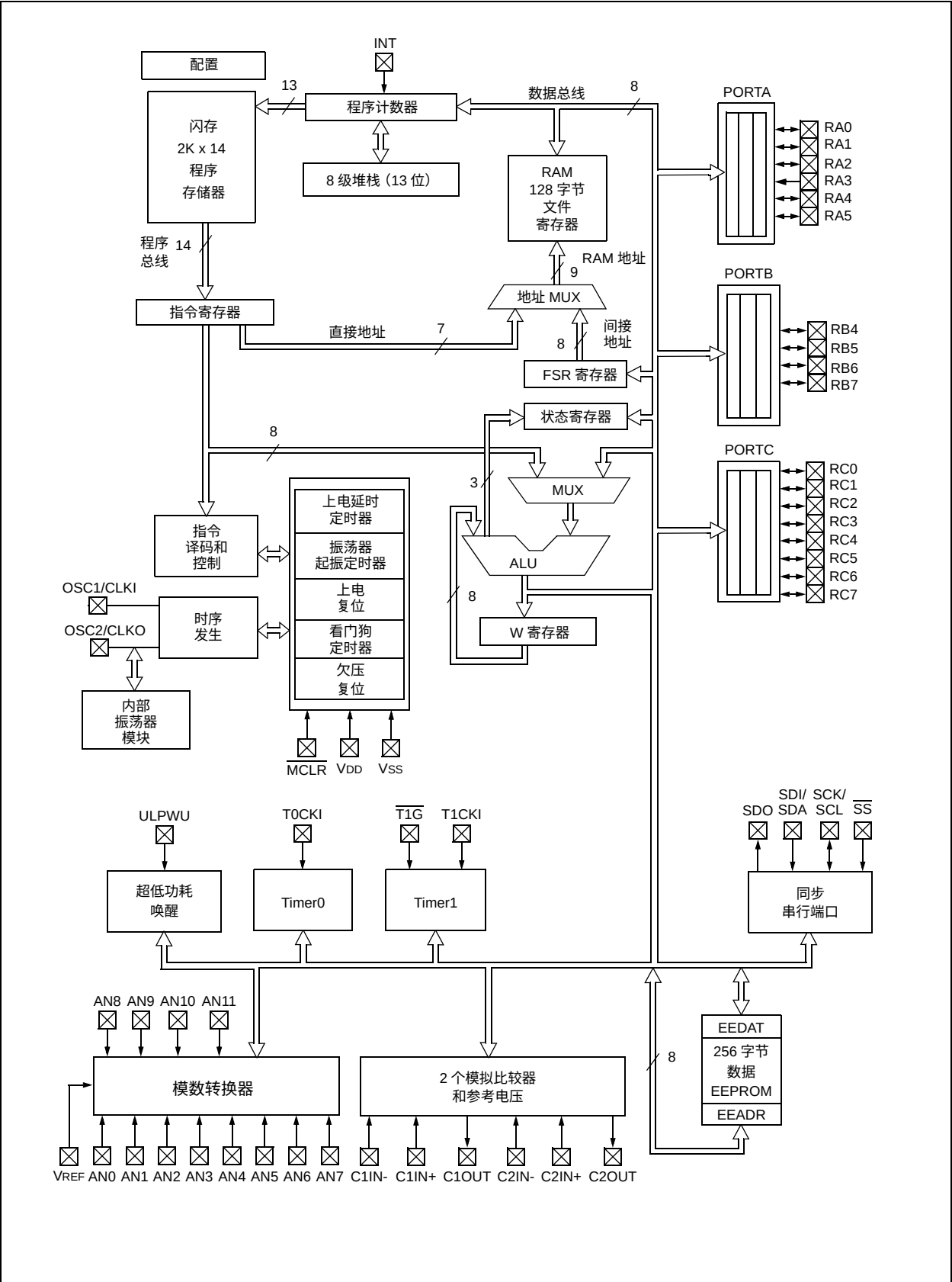
图 1-2 : PIC16F677 框图
