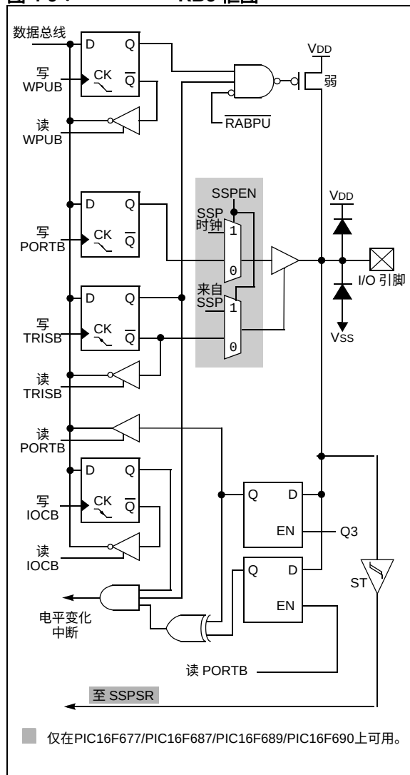
图 4-9： RB6 框图
