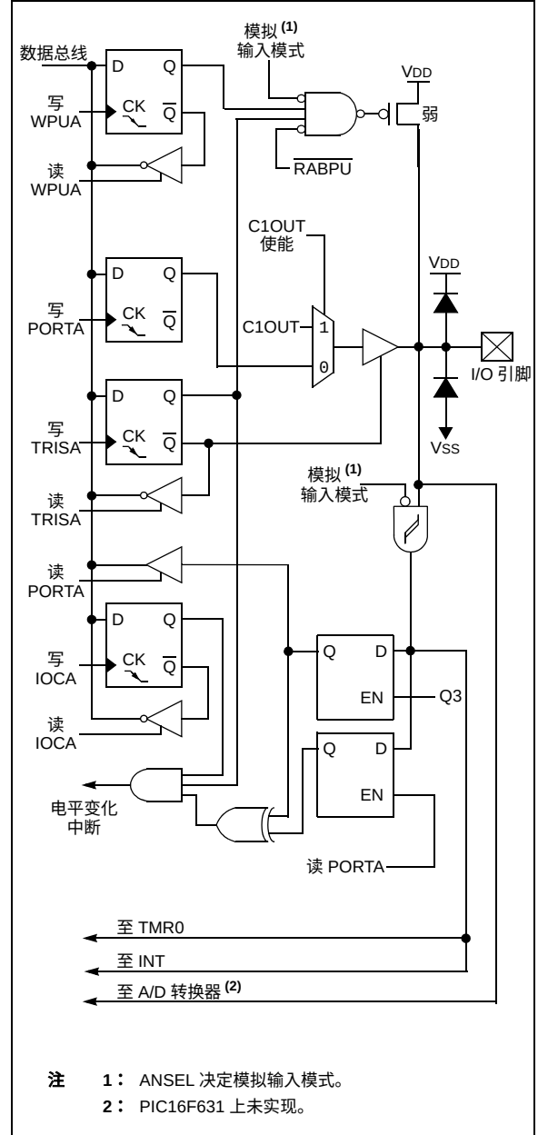
图 4-3： RA2 框图
