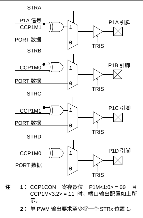
图 11-18：转向的简化框图
