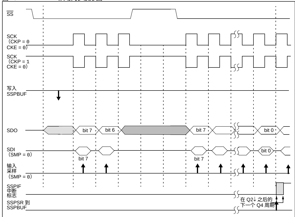
图 13-4： 从同步波形图
