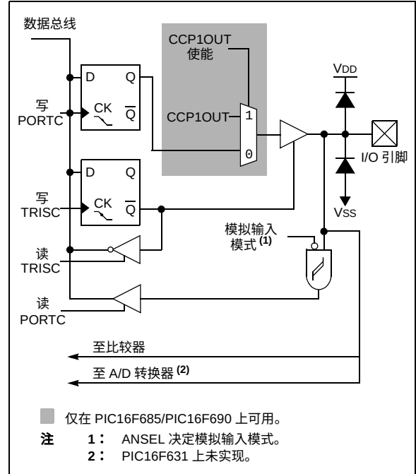
图 4-12： RC2 和 RC3 框图
