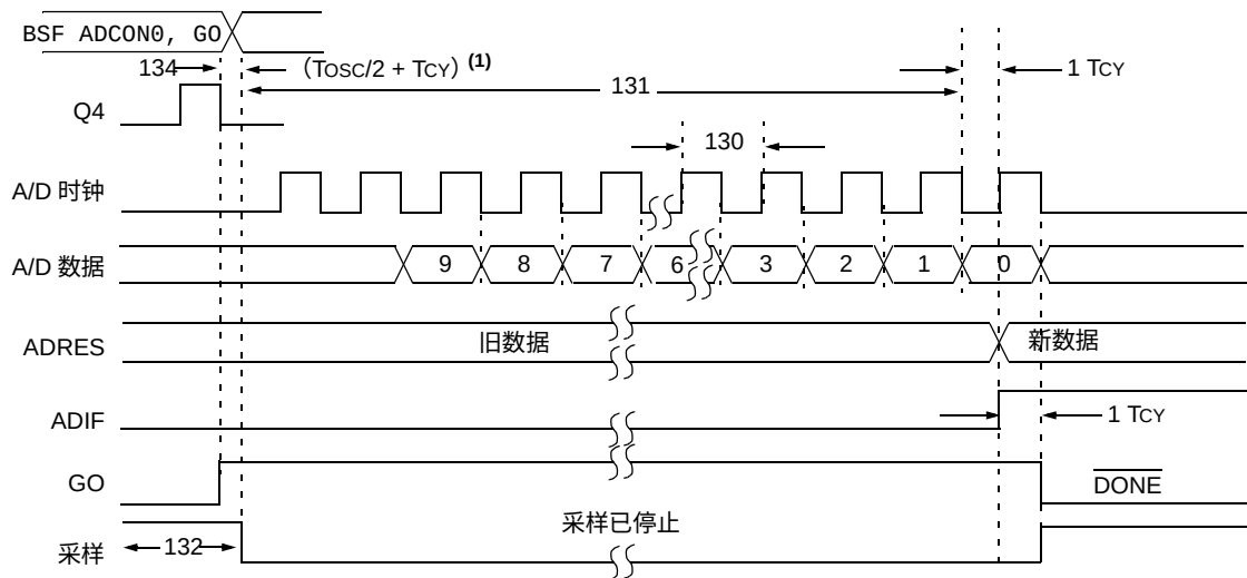
图 17-19： A/D 转换时序（休眠模式）
