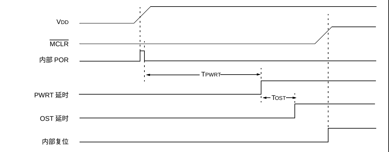
图 14-5：上电时的延时时序（MCLR 延时）：情形 2
