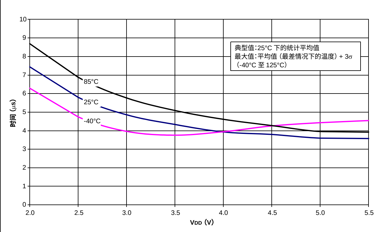
图 18-34：不同温度的最小 HFINTOSC 起振时间－V DD 曲线
