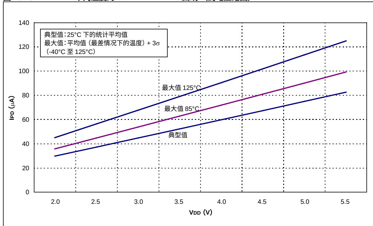
图 18-20：不同温度的 CVREF IPD — VDD 曲线（高电压范围）
