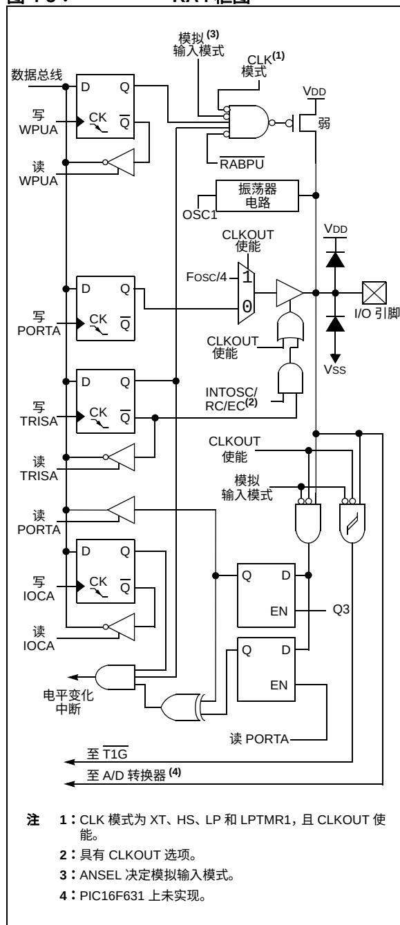
图 4-5： RA4 框图
