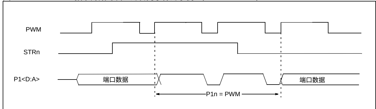
图 11-20： 指令开始时发生的转向事件的示例 (STRSYNC = 1)
