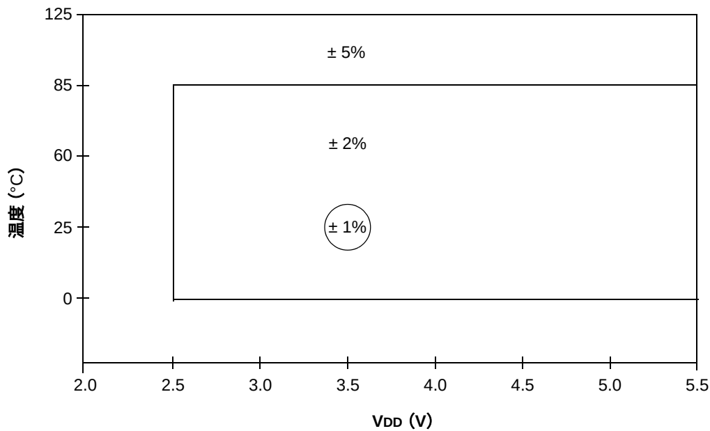
图 17-2： 器件 VDD 和温度范围内 HFINTOSC 的频率精度
