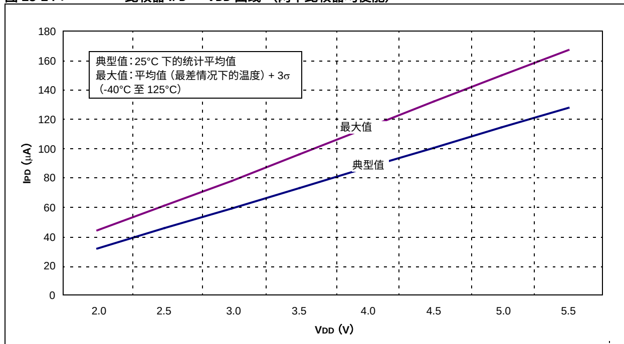
图 18-14： 比较器 IPD – VDD 曲线（两个比较器均使能）
