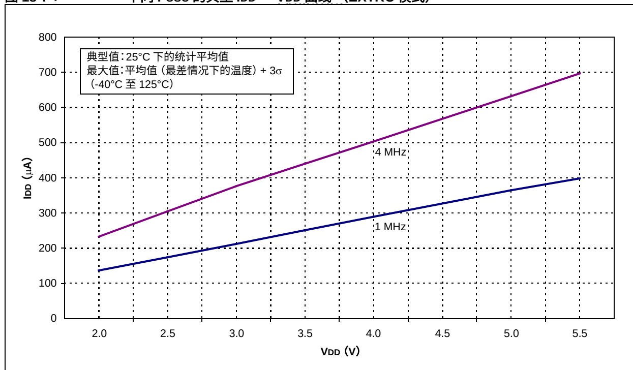
图 18-7：不同 Fosc 的典型 I DD - V DD 曲线（EXTRC 模式）
