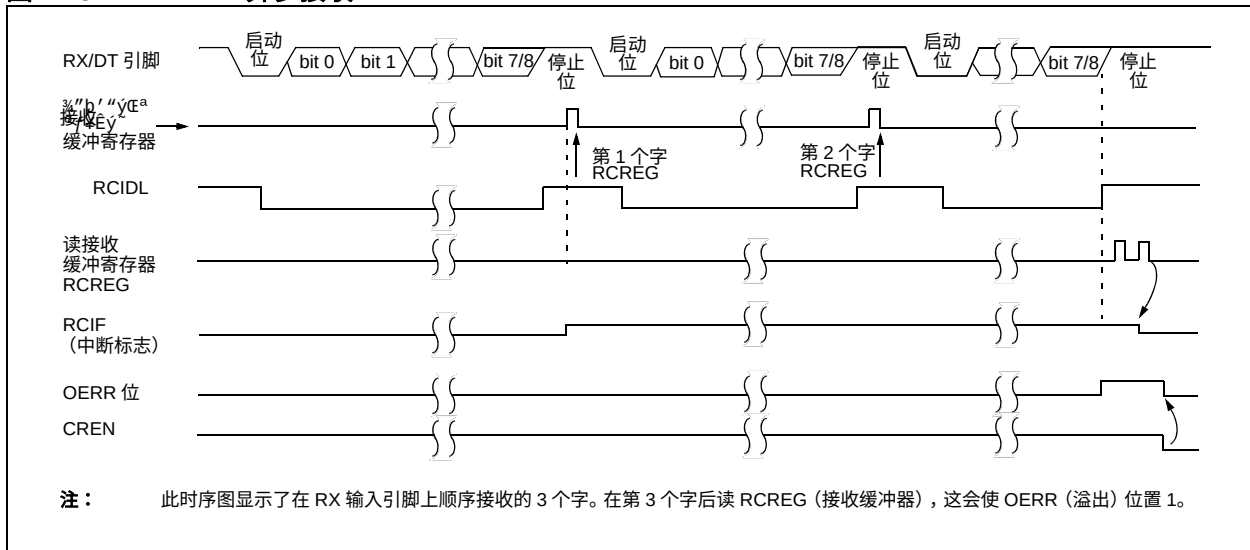
图 12-5： 异步接收
