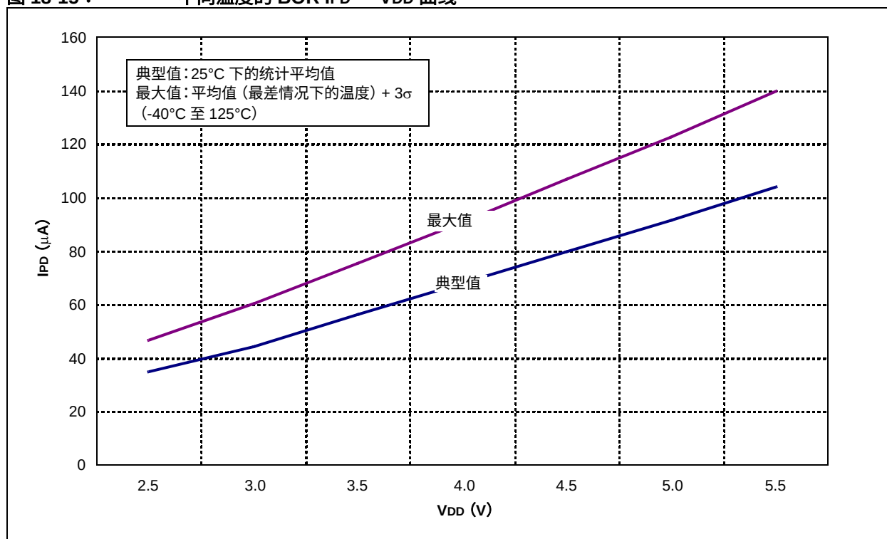
图 18-15： 不同温度的 BOR IPD – VDD 曲线
