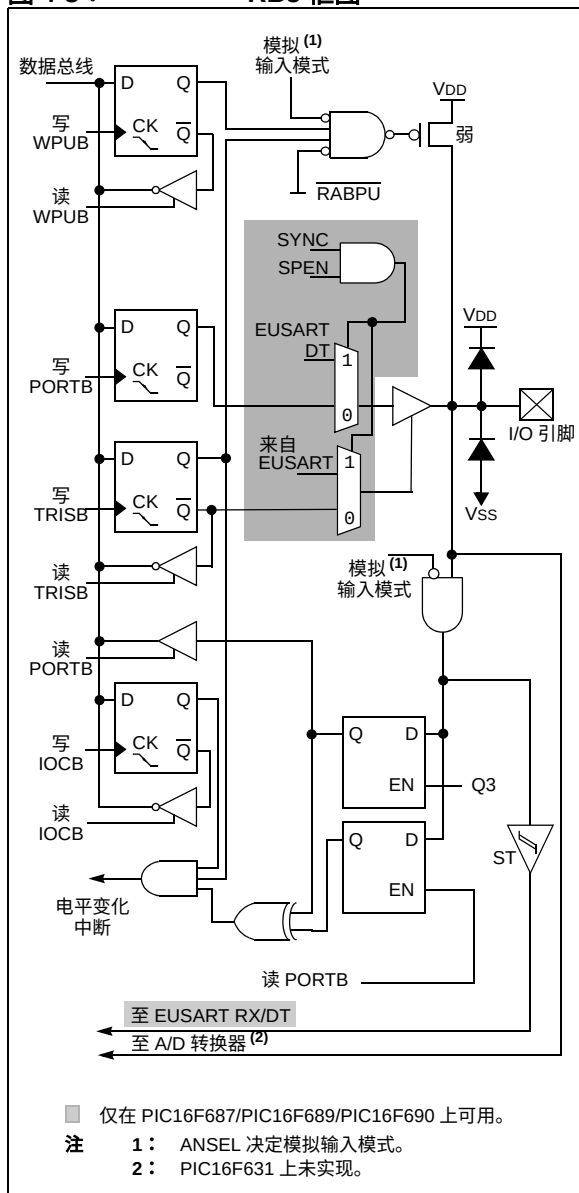
图 4-8： RB5 框图
