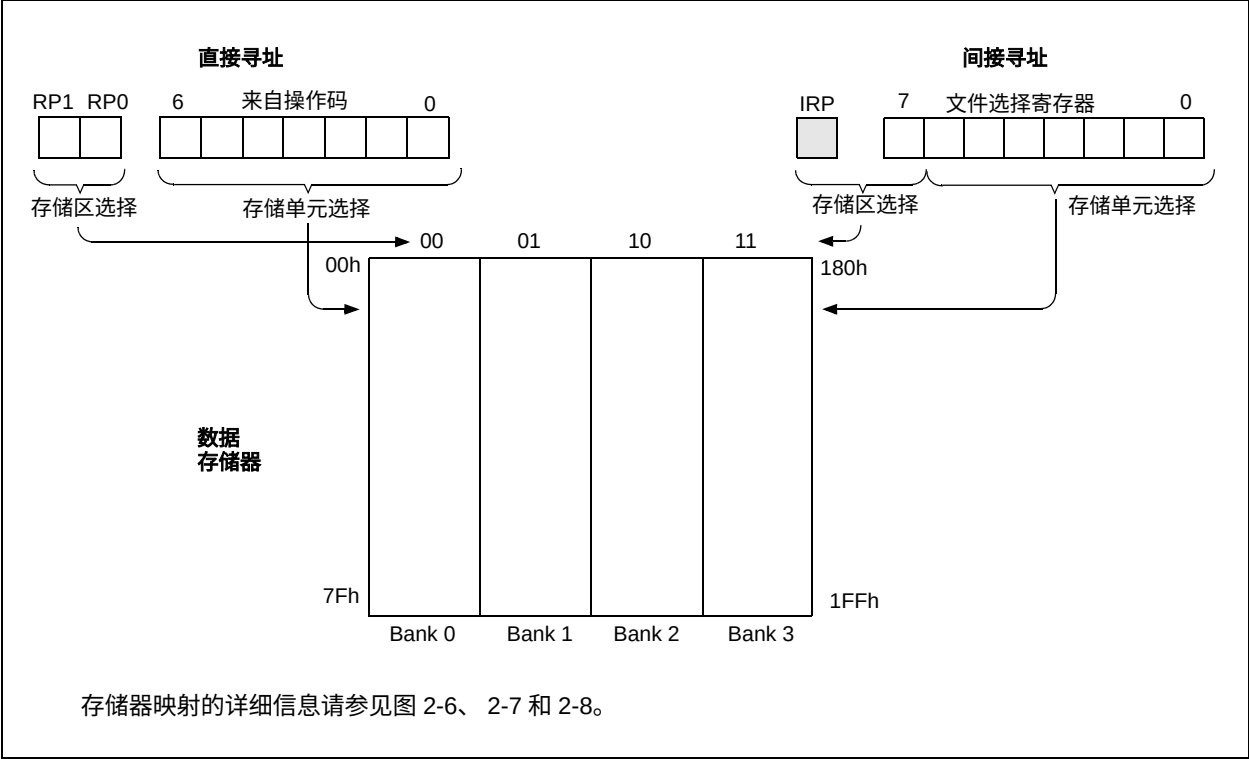
图 2-10： PIC16F631/677/685/687/689/690 的直接 / 间接寻址
