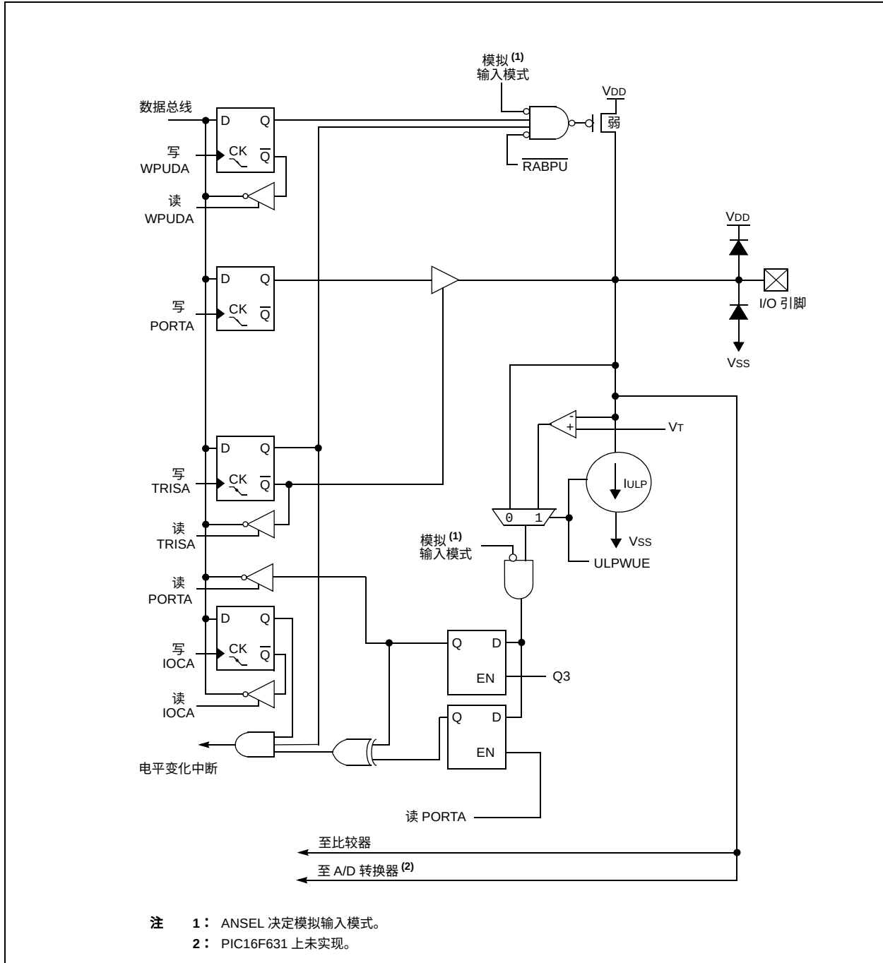
图 4-1： RA0 框图
