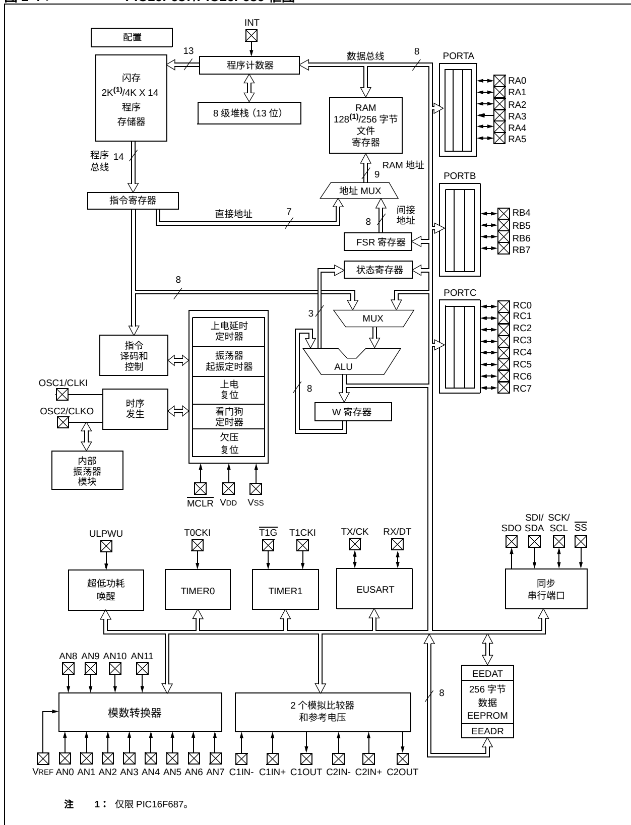
图 1-4 : PIC16F687/PIC16F689 框图
