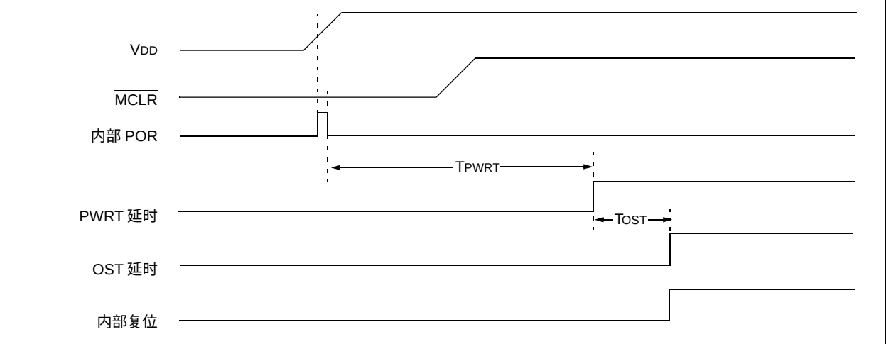
图 14-4：上电时的延时时序（MCLR 延时）：情形 1
