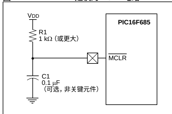
图 14-2： 建议的 \overline{\text{MCLR}} 电路
