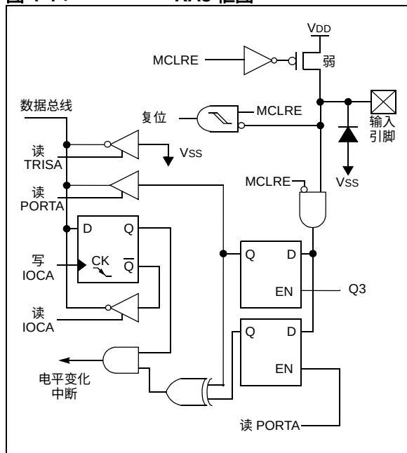
图 4-4: RA3 框图
