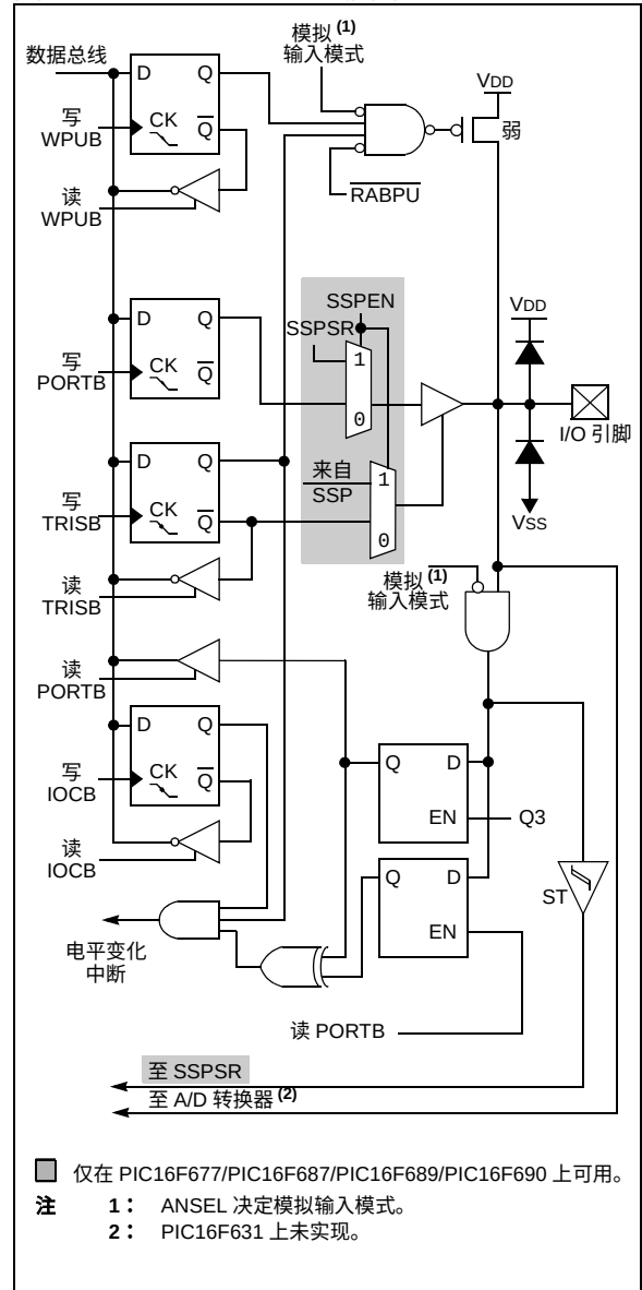
图 4-7： RB4 框图
