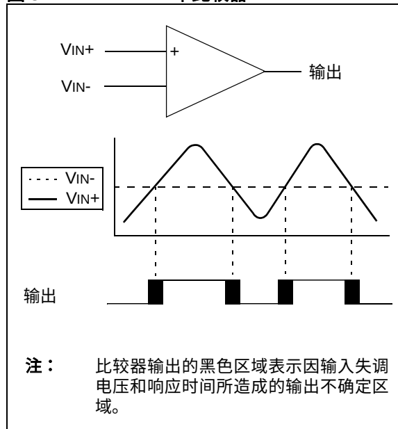
图 8-1： 单比较器
