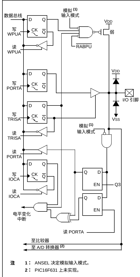
图 4-2： RA1 框图
