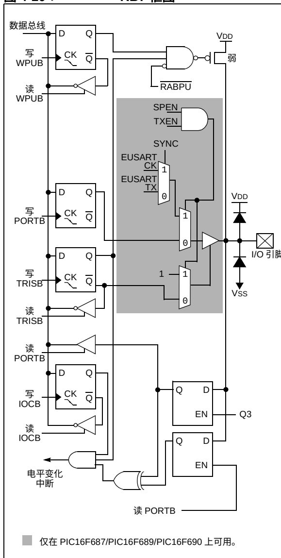
图 4-10： RB7 框图
