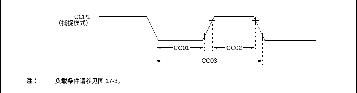
图 17-9： 捕捉 / 比较 / PWM 时序 (ECCP)
