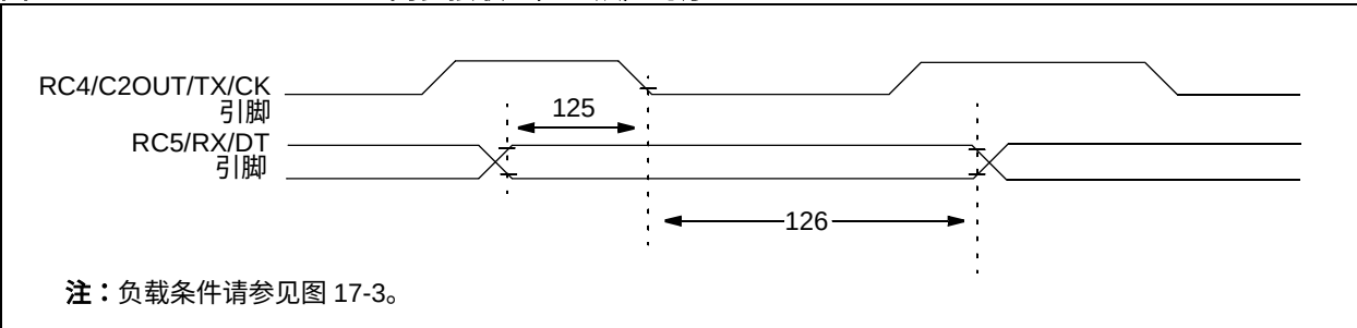
图 17-11： EUSART 同步接收（主 / 从）时序
