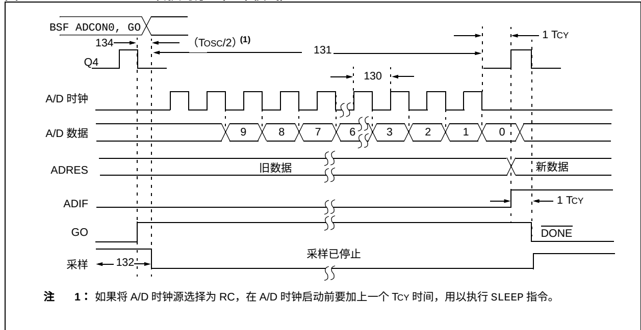
图 17-18： A/D 转换时序（正常模式）
