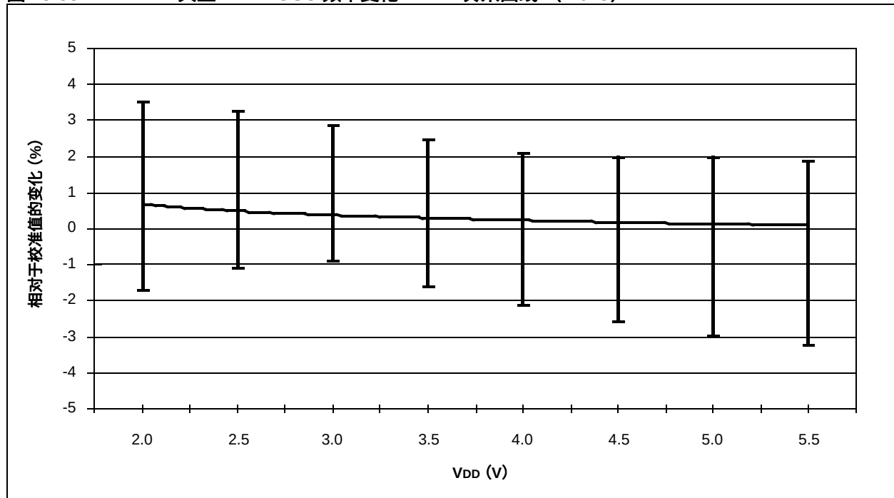
图 18-38 : 典型 HFINTOSC 频率变化— V_{DD} 关系曲线 ( -40^{\circ}\text{C} )
