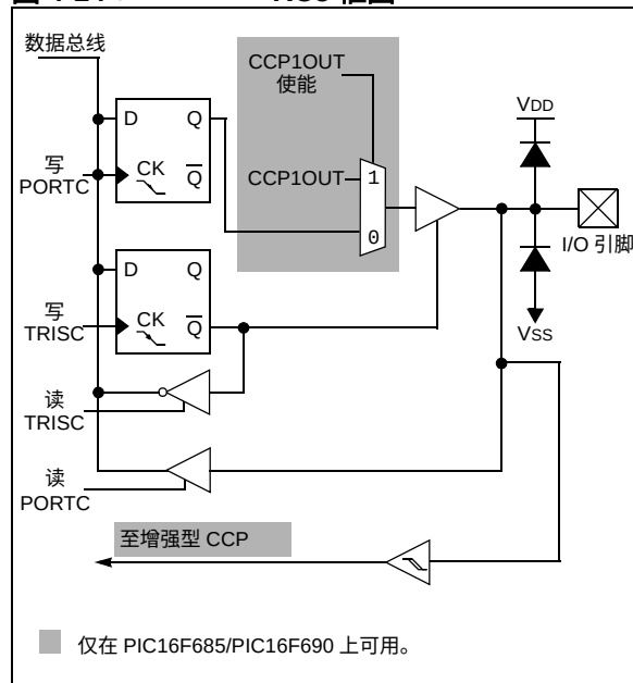
图 4-14： RC5 框图
